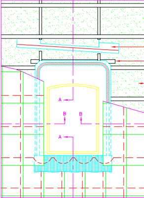
Visat vinkelrikt på tak 1:20
